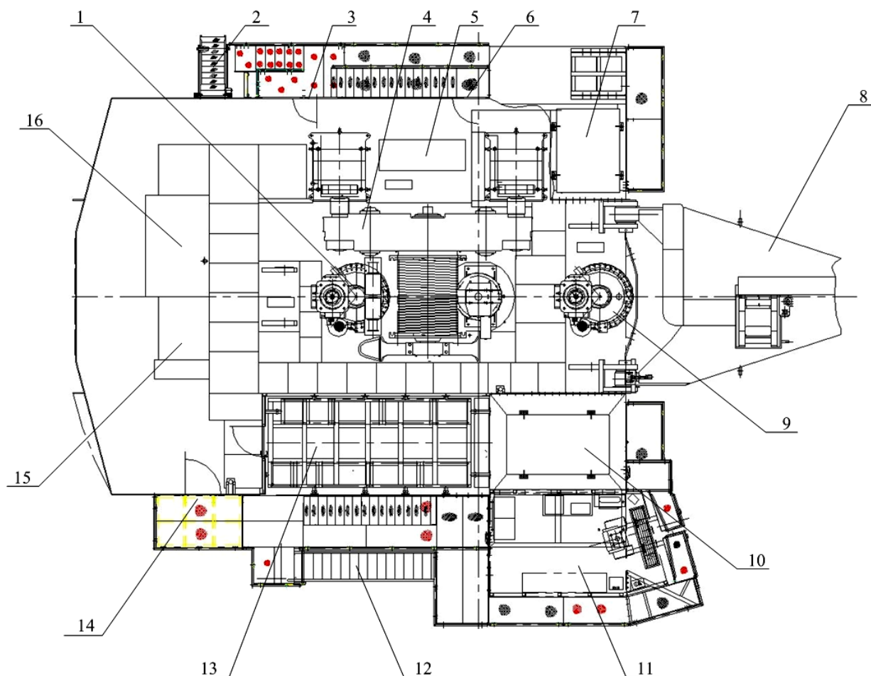
Рисунок 2. Расположение оборудования на поворотной платформе
